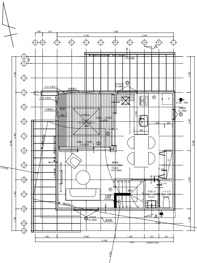
2階平面図
