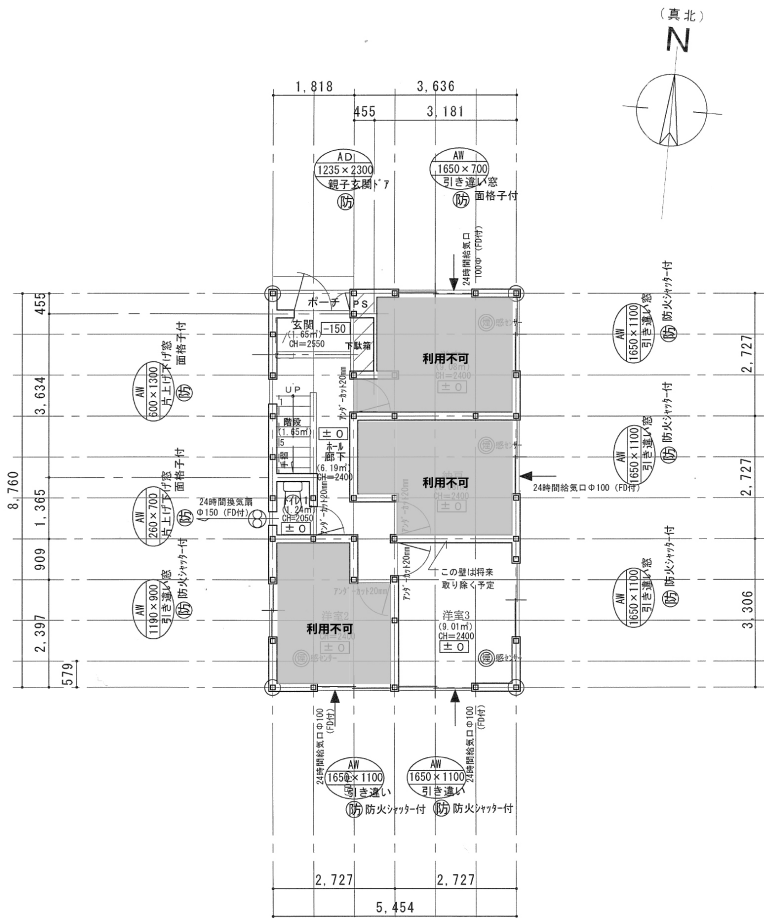
1 階平面図
