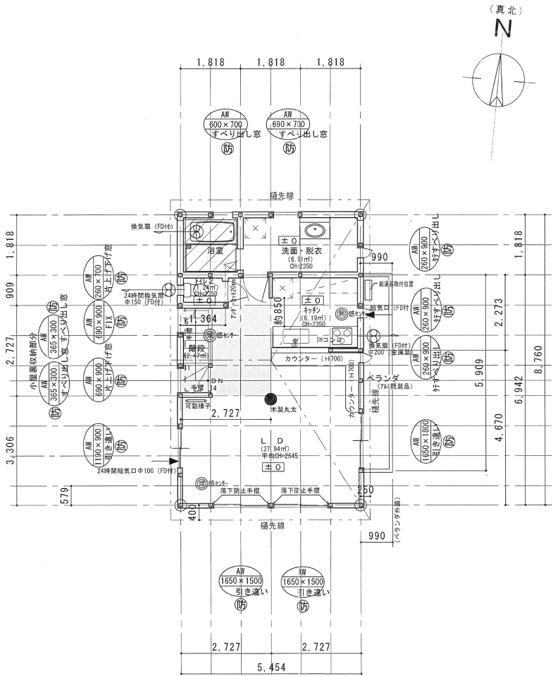
1 階平面図
